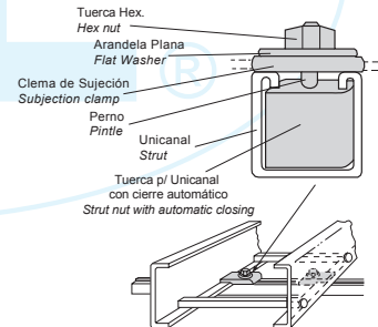
Diagrama: Tuercas con Clema de Sujeción Diagram: Nut subsection clamp
