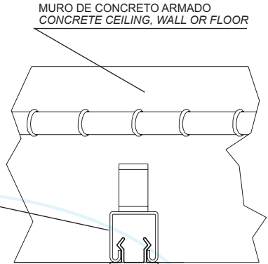
UNICANAL CON INSERTOS CONCRETE INSERT STRUT
